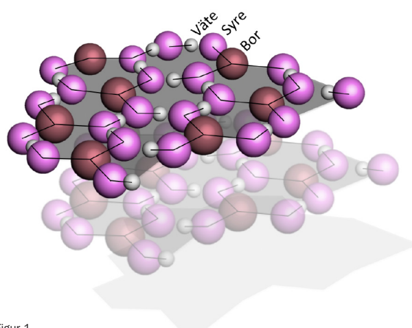
Figur 1 Borsyra har en lagrad struktur. Varje lager består av plana borsyrakärl med starka bindningar mellan atomerna medan de är svaga bindningar mellan lagren. Detta gör att de glider lätt mot varandra.
