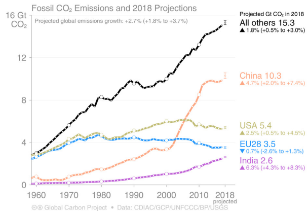
Figur 2: Fossila CO 2 -utsläpp och prognos för 2018; orange: Kina, grön: USA, blå: EU28, lila: Indien, svart: Alla övriga 7
