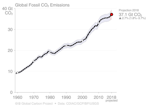
Figur 1: Globala fossila CO 2 -utsläpp, texten till kurvan anger Prognos för 2018 2
